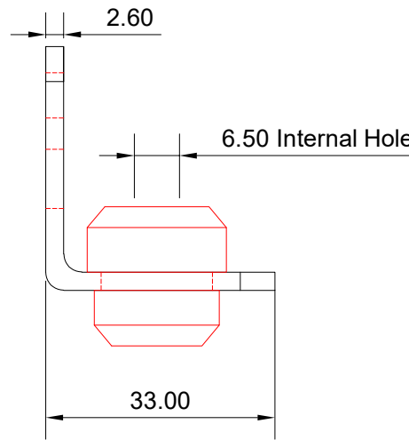
Elevation Scale 1:1
