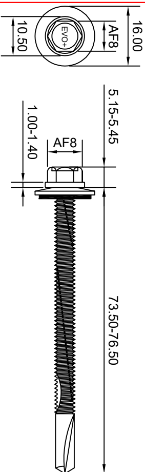
BMW5.5-75-5
