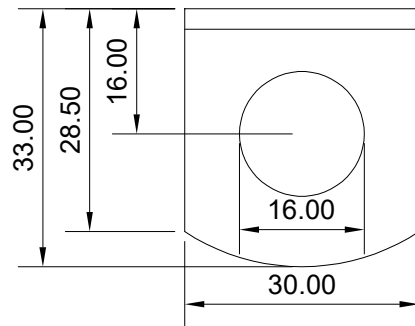
Plan Scale 1:1
