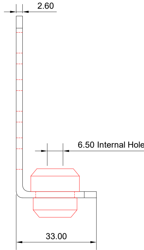
Elevation Scale 1:1
